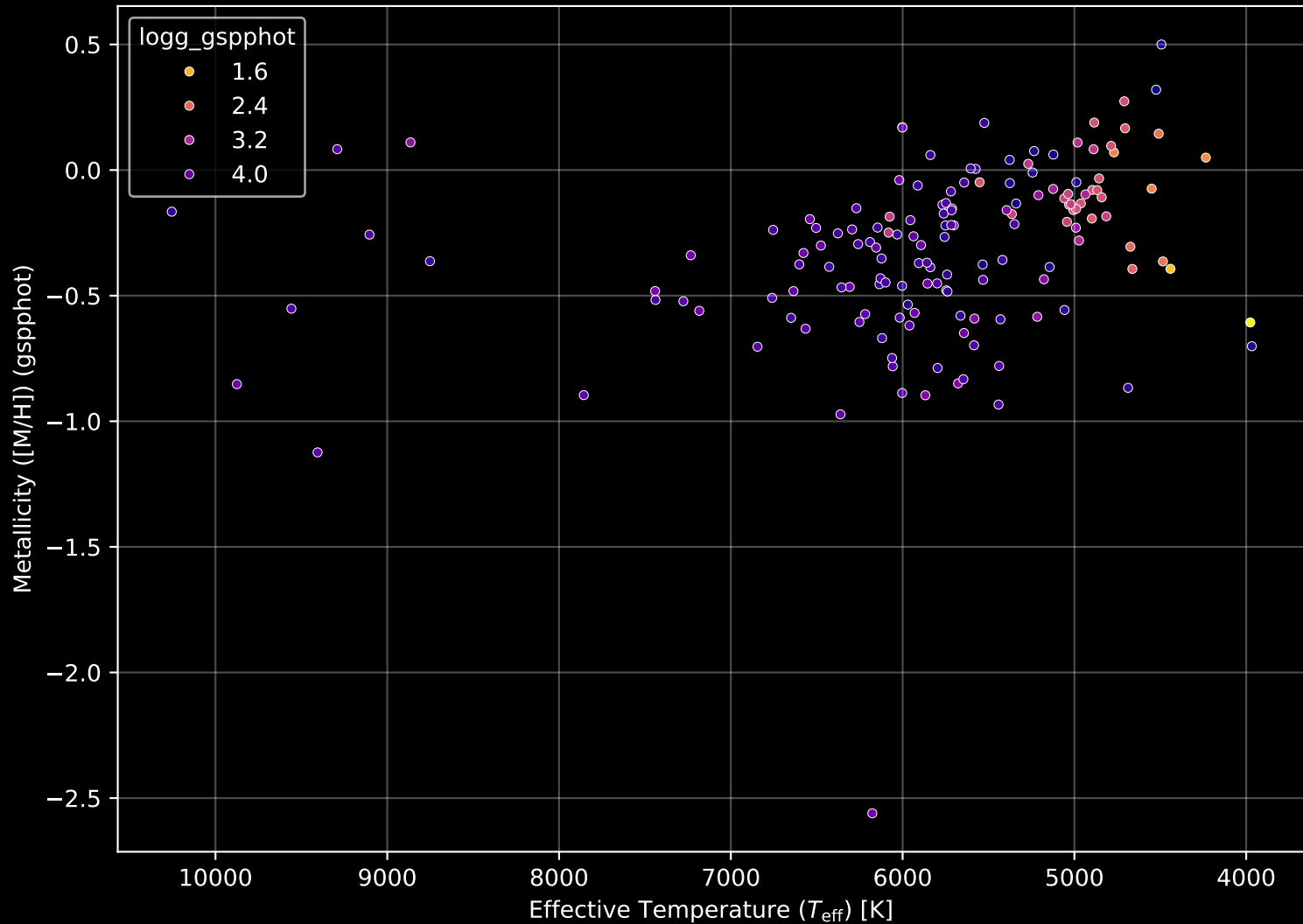
GALAH DR4 Field: [7168] Stellar Population Parameters (n= 154)
