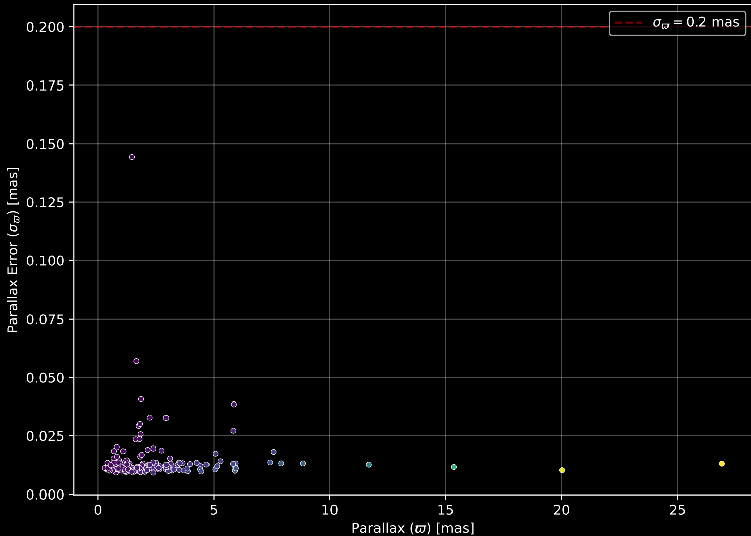
GALAH DR4 Field: [7168] Parallax Quality (n= 154)
