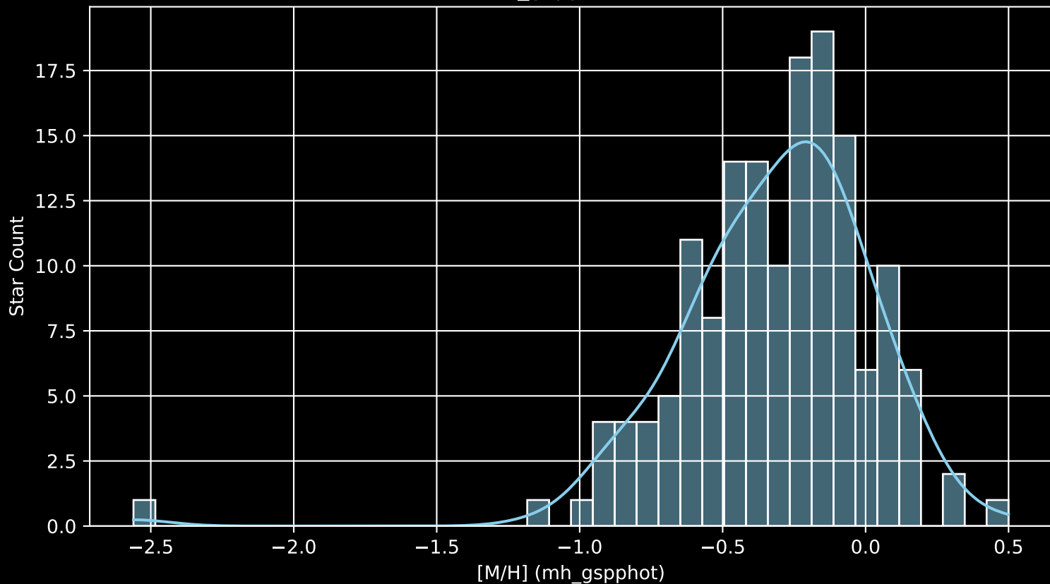
GALAH DR4 Field: [7168] [M/H] (mh_gspphot) (n= 154)
